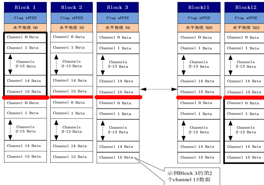
图 6.1 单回波数据块结构
