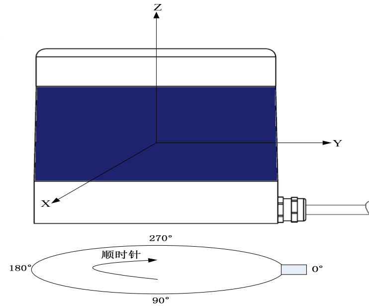
图 1.3 C16 激光雷达坐标系和扫描方向
