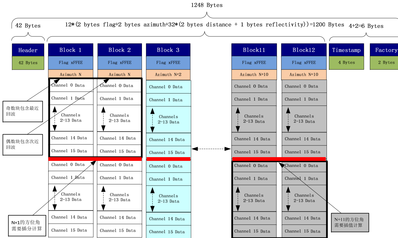
图 4.2 C16 双回波数据格式
