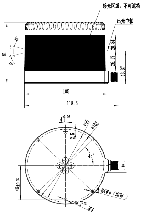
图 1.1 C16 小型激光雷达的结构尺寸图
