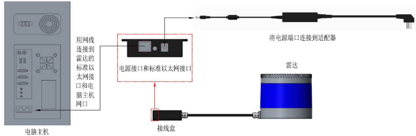
图 3.1 连接雷达和电脑
