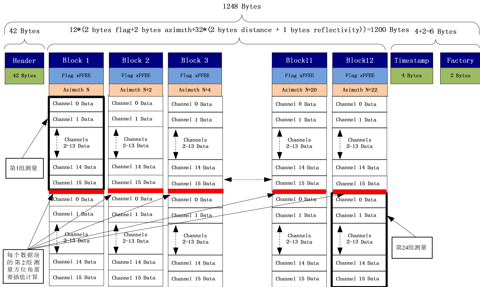
图 4.1 C16 单回波数据格式
